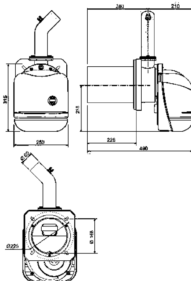
pav. 11 — Matmenys SUN P12
