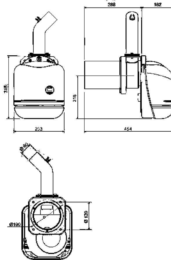
pav. 10 — Matmenys SUN P7
